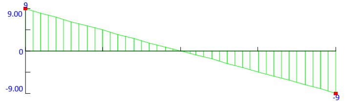
Shear Diagram (Y) (kip)
